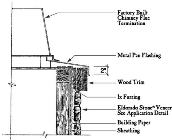
CHIMNEY CAP
