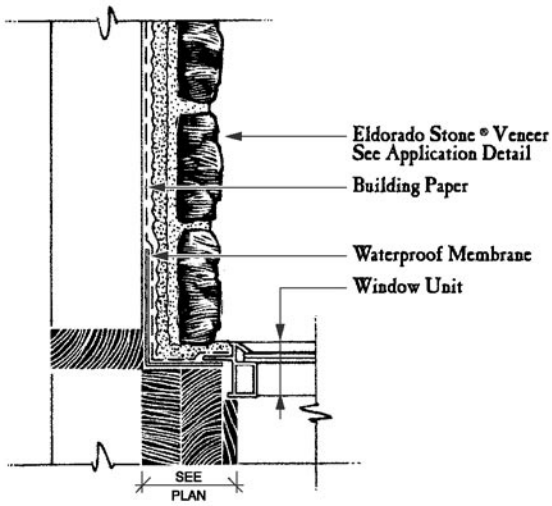
WINDOW JAMB
