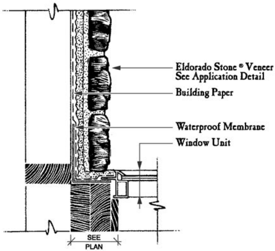
WINDOW JAMB
