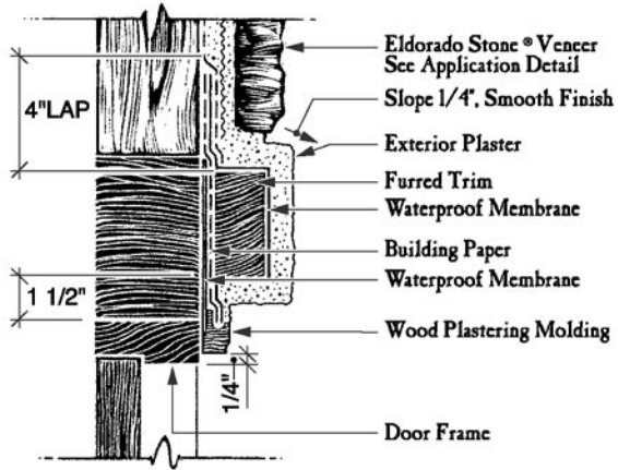
DOOR HEADER Trim Furred
